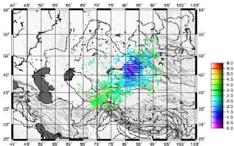
Рисунок 5. Карта минимальных магнитуд сейсмических событий, зарегистрированных станцией PS23-Мақанчи по данным оперативного бюллетеня ЦСОССИ за 2003 г
